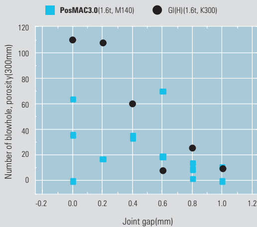
기공결함과 이음부 Gap 간격의 관계
