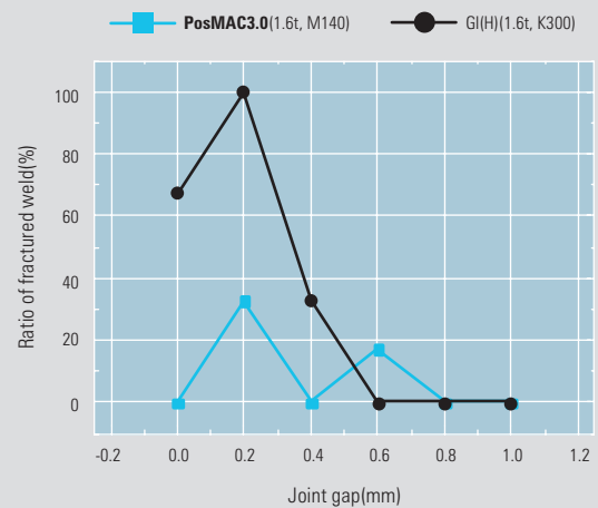
용접부 파단율과 이음부 Gap 간격의 관계
